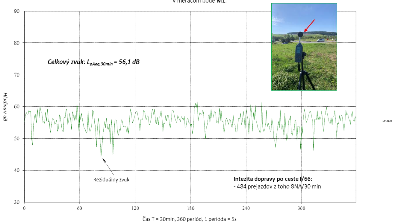
Obr. 3.4 Informatívny časový priebeh ekvivalentných hladín hluku L_{pAeq,5s} v čase T = 30 min. od 08:00 hod. do 08:30 hod. zo dňa 30.04.2024 v meracom bode M1.
