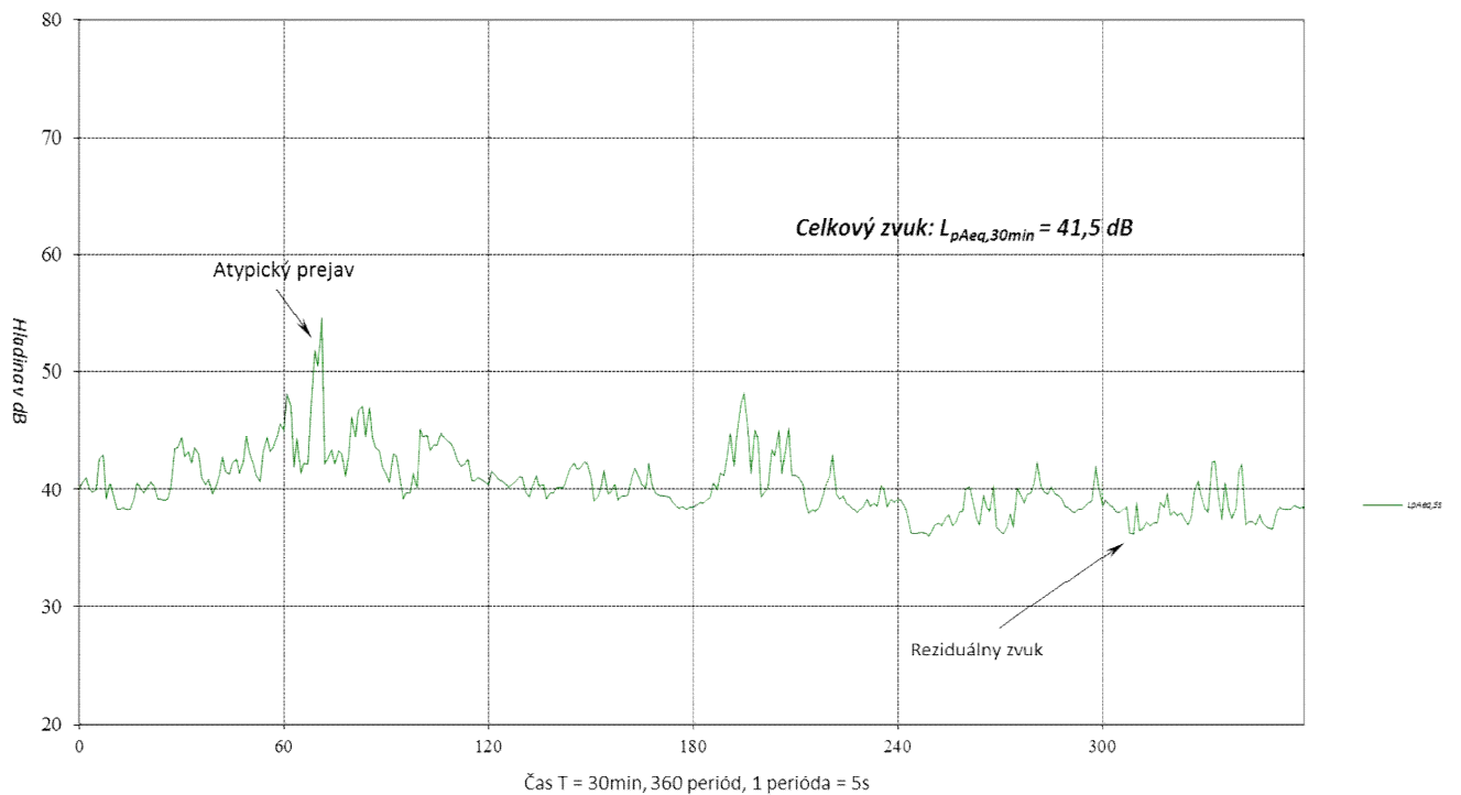
Obr. 3.6 Informatívny časový priebeh ekvivalentných hladín hluku L_{pAeq,5s} v čase T = 30 min. od 23:15 hod. do 23:45 hod. zo dňa 30.04.2024 v meracom bode M1.
