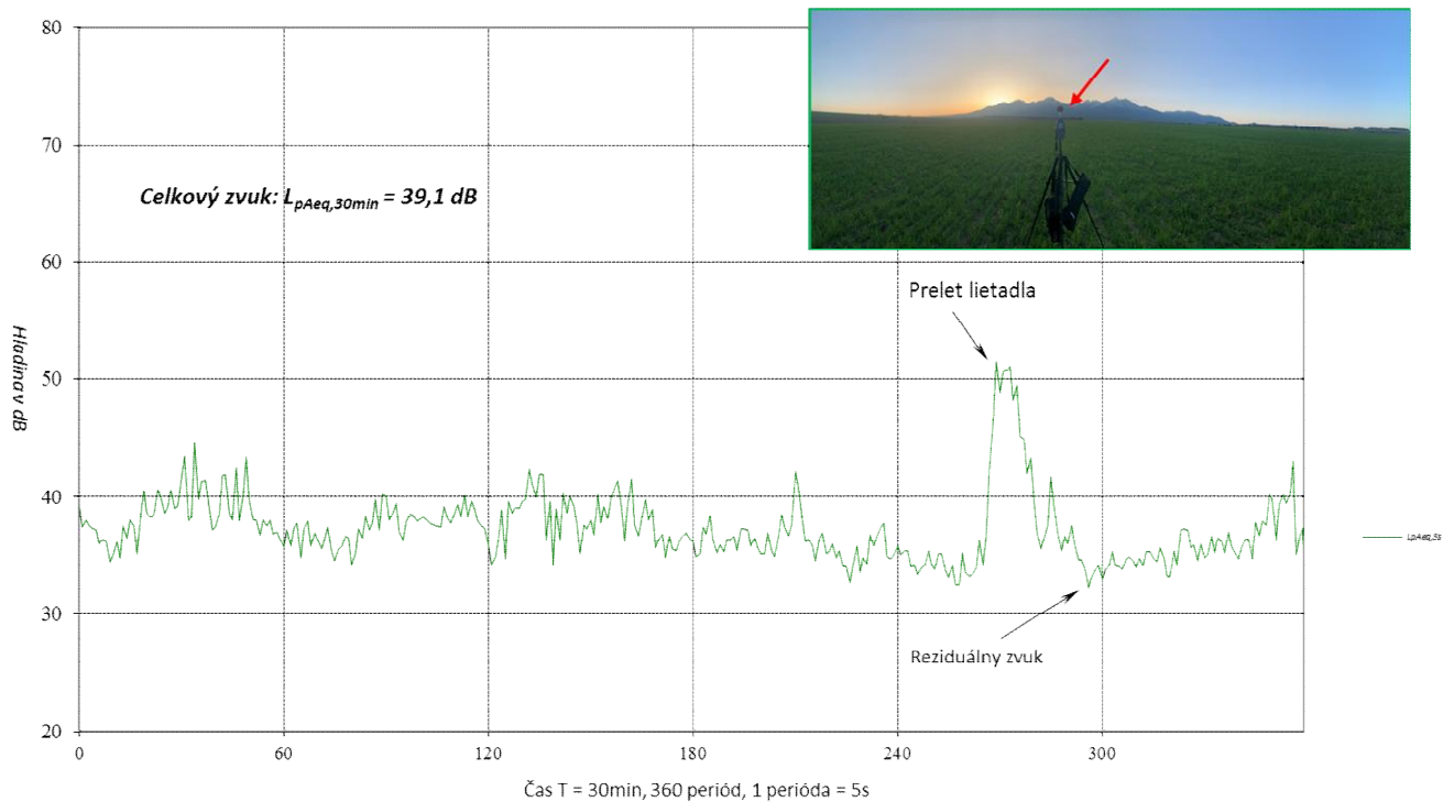
Obr. 3.8 Informatívny časový priebeh ekvivalentných hladín hluku L_{pAeq,5s} v čase T = 30 min. od 18:00 hod. do 18:30 hod. zo dňa 30.04.2024 v meracom bode M2.
