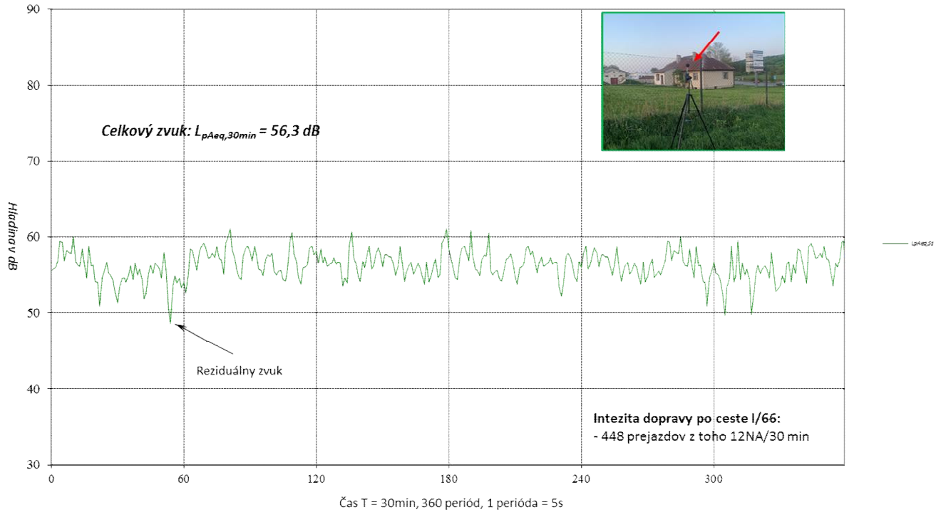
Obr. 3.5 Informatívny časový priebeh ekvivalentných hladín hluku L_{pAeq,5s} v čase T = 30 min. od 18:50 hod. do 19:20 hod. zo dňa 30.04.2024 v meracom bode M1.
