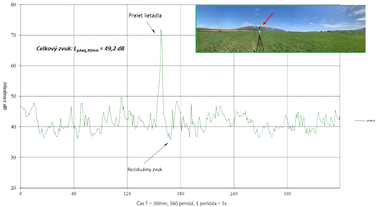
Obr. 3.7 Informatívny časový priebeh ekvivalentných hladín hluku L_{pAeq,5s} v čase T = 30 min. od 8:45 hod. do 09:15 hod. zo dňa 30.04.2024 v meracom bode M2.
